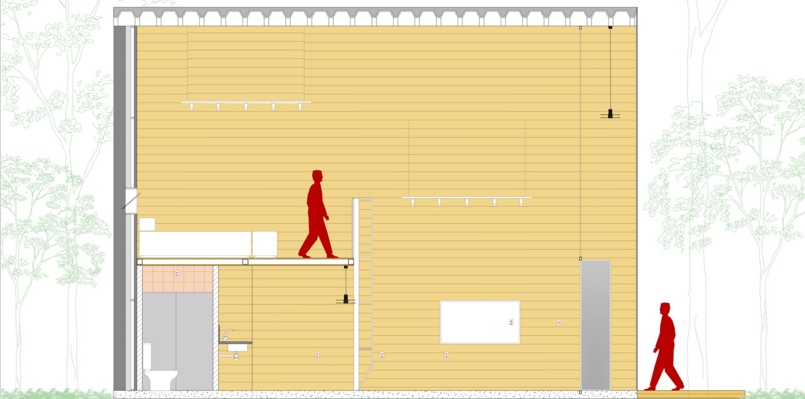
CORTE B
